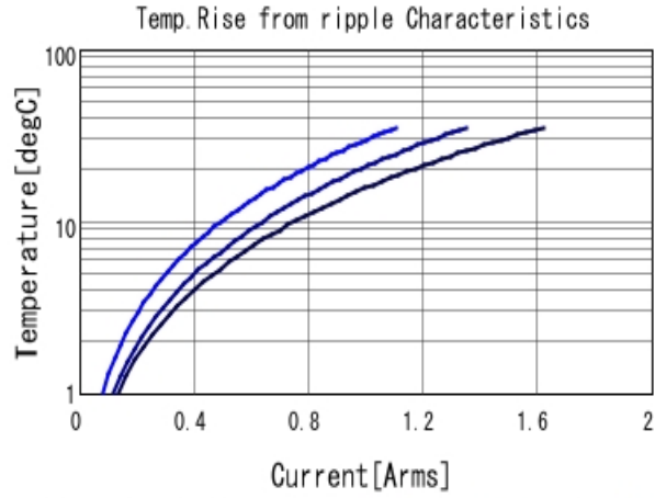
GRT155C81E224KE01 Temp. rise ■ 300kHz ■ 600kHz ■ 1MHz
