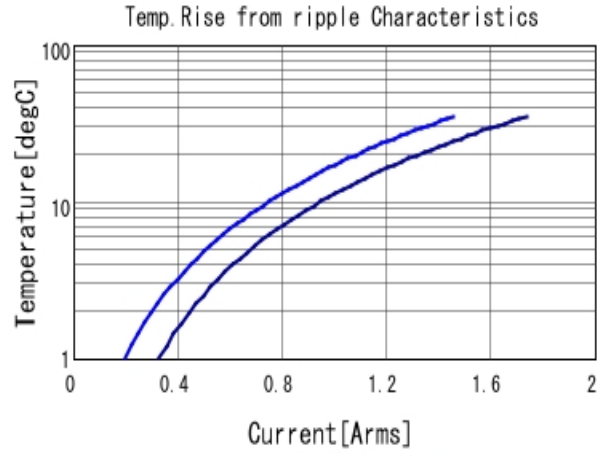
■ GRT033C80J224KE01 Temp. rise ■ 600kHz ■ 1MHz
