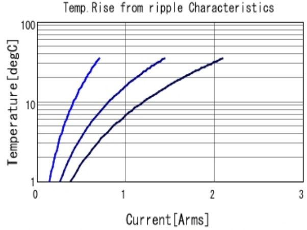
GRM43DR72E334KW01 Temp. rise ■ 30kHz ■ 100kHz ■ 300kHz
