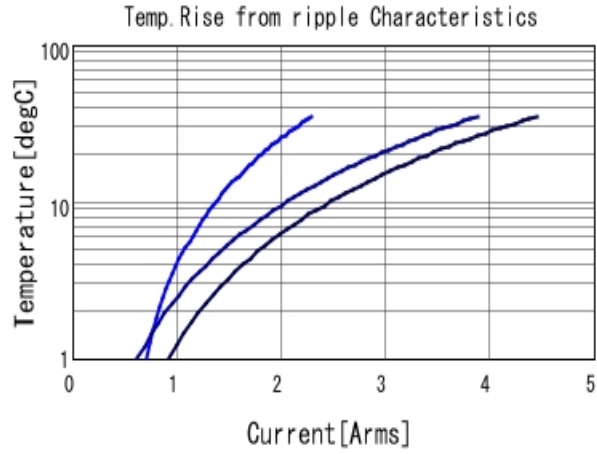
GRM32RR71H105KA01 Temp. rise ■ 100kHz ■ 500kHz ■ 1MHz
