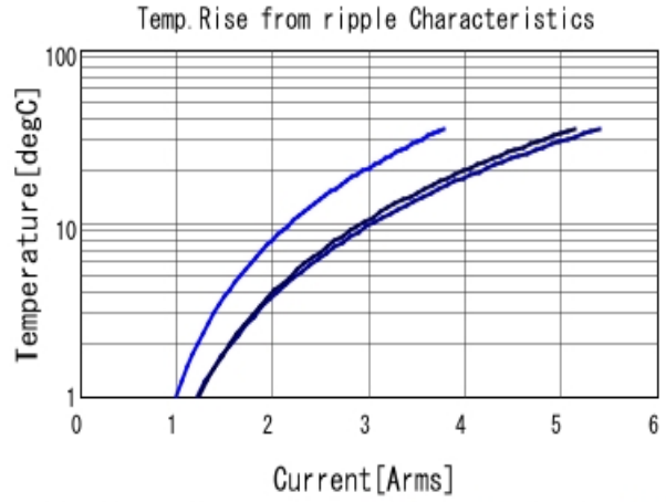
GRM32ER72A225KA35 Temp. rise ■ 100kHz ■ 500kHz ■ 1MHz
