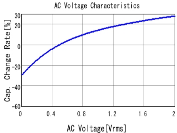
■ GRM32ER71E226KE15 C-AC Voltage capchange, DCOV, 25.0d
