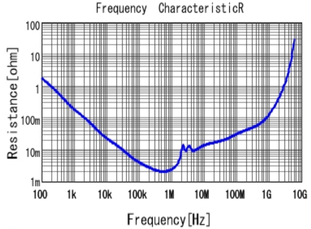
■ GRM32ER71E226KE15 R DCOV, 25degC
