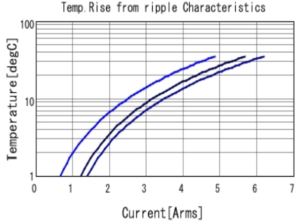
GRM32ER71E226KE15 Temp. rise ■ 80kHz ■ 400kHz ■ 800kHz
