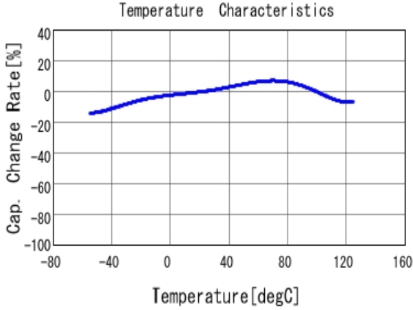
■ GRM32ER71E226KE15 C-Temp. capchange, DCO. 0V, ACO. 5V rm
