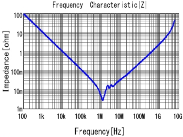
■ GRM32ER71E226KE15 |Z| DCOV, 25degC
