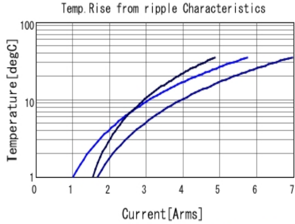
GRM32ER61E226KE15 Temp. rise ■ 80kHz ■ 400kHz ■ 800kHz
