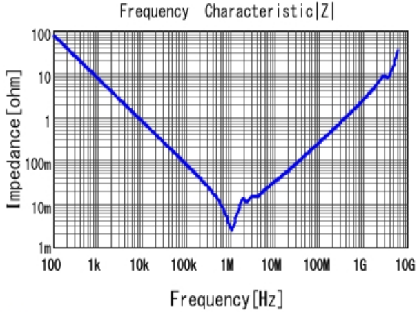
■ GRM32ER61E226KE15 |Z| DCOV, 25degC
