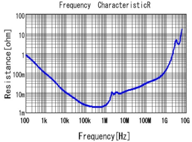
■ GRM32ER61E226KE15 R DCOV, 25degC
