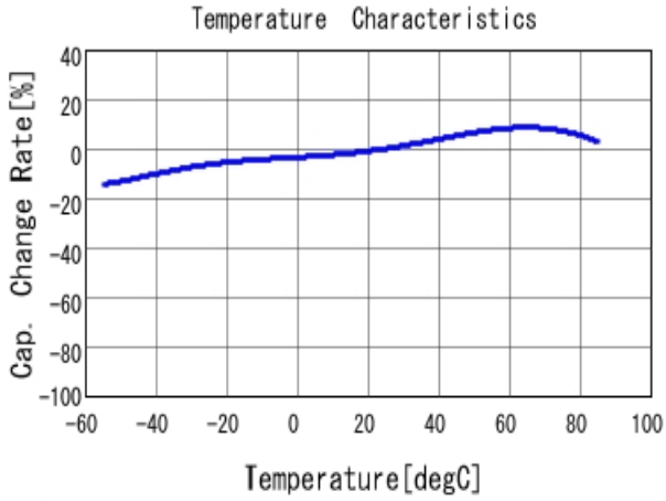
■ GRM32ER61E226KE15 C-Temp. capchange, DCO. 0V, ACO. 5V rm
