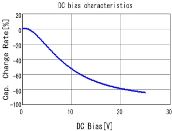
■ GRM32ER61E226KE15 C-DC bias capchange, 25.0degC, AC0.
