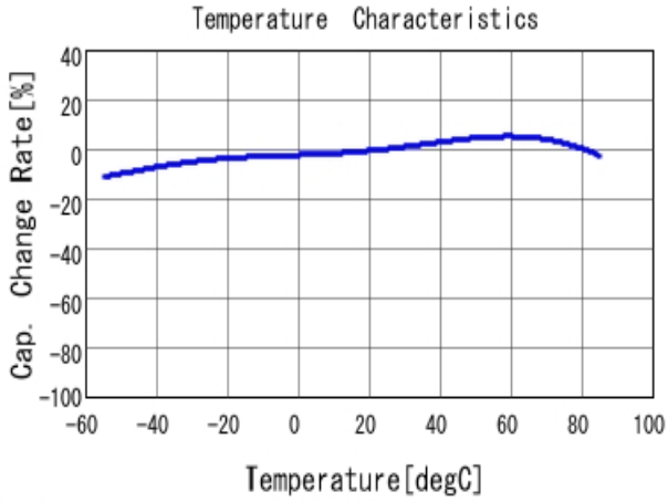
■ GRM32ER61C476KE15 C-Temp. capchange, DCO. 0V, ACO. 5V rm
