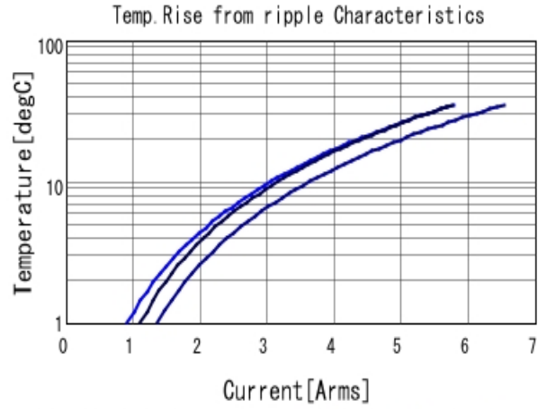
GRM32ER61C476KE15 Temp. rise ■ 60kHz ■ 300kHz ■ 600kHz
