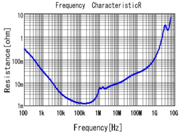
■ GRM32ER60J107ME20 R DCOV, 25degC
