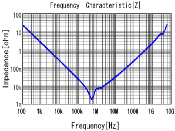
■ GRM32ER60J107ME20 |Z| DCOV, 25degC
