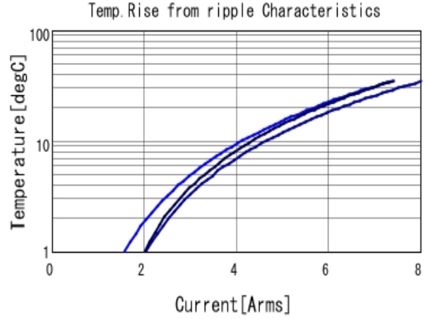
GRM32ER60J107ME20 Temp. rise ■ 50kHz ■ 200kHz ■ 400kHz
