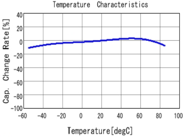
■ GRM32ER60G337ME05 C-Temp. capchange, DCO. 0V, ACO. 15Vr
