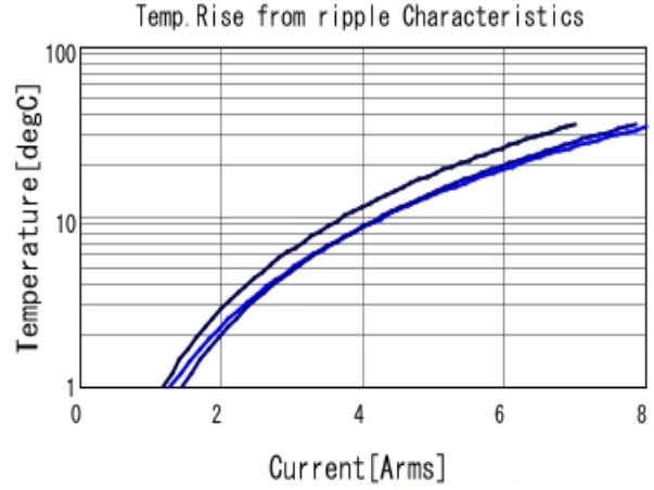
GRM32ER60G337ME05 Temp. rise ■ 50kHz ■ 200kHz ■ 400kHz
