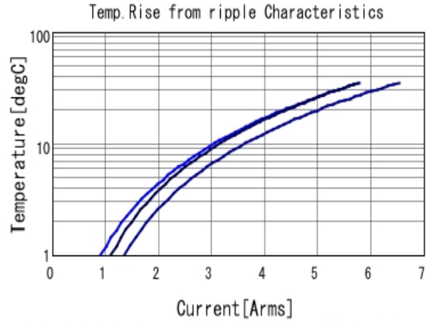
GRM32EC81C476KE15 Temp. rise ■ 60kHz ■ 300kHz ■ 600kHz
