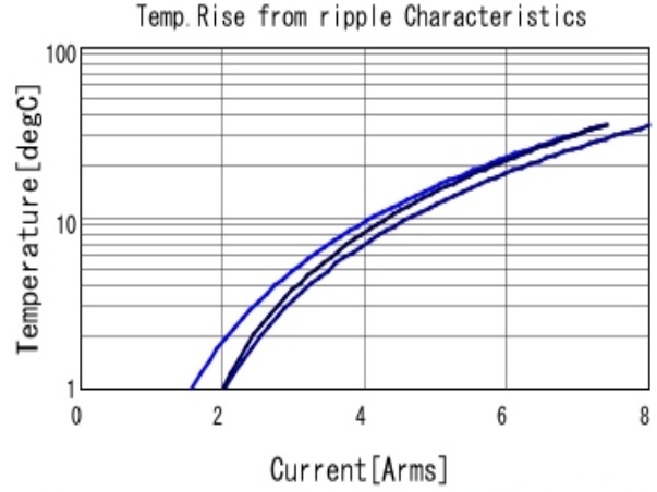
GRM32EC80J107ME20 Temp. rise ■ 50kHz ■ 200kHz ■ 400kHz
