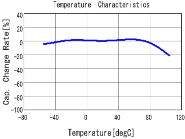
■ GRM32EC80J107ME20 C-Temp. capchange, DCO. 0V, ACO. 5V rm
