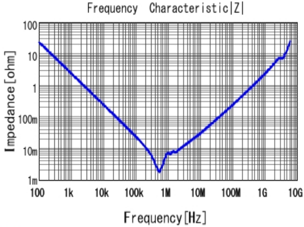
■ GRM32EC80J107ME20 |Z| DCOV, 25degC
