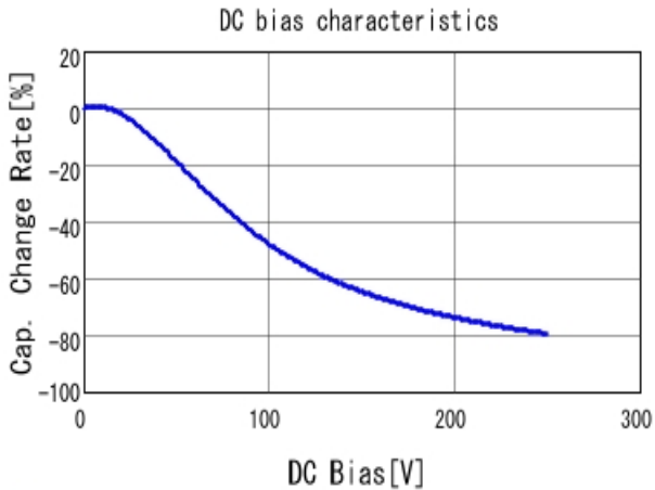
■ GRM32DR72E224KW01 C-DC bias capchange, 25.0degC, AC1V
