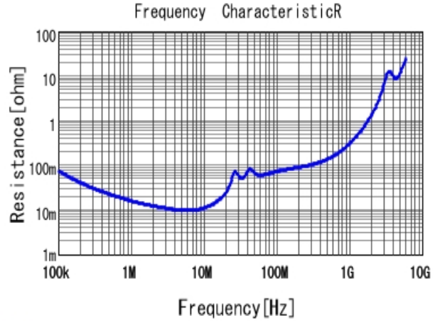
■ GRM32DR72E224KW01 R DCOV, 25degC
