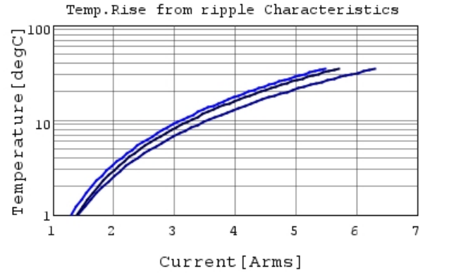
GRM32DR61E106KA12 Temp.rise 80kHz
