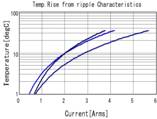
GRM32DC72A475KE01 Temp. rise ■ 100kHz ■ 500kHz ■ 1MHz
