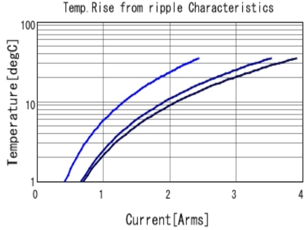
GRM31MR72A684KA35 Temp. rise ■ 200kHz ■ 500kHz ■ 1MHz
