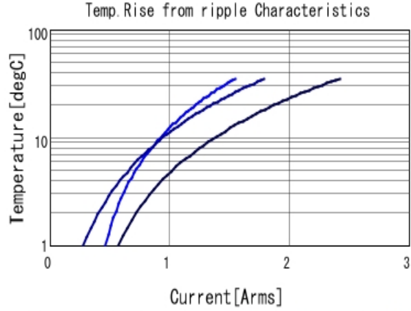
GRM31MR72A224KA01 Temp. rise ■ 300kHz ■ 600kHz ■ 1MHz
