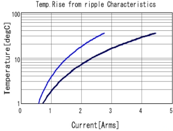
GRM31MR71E225KA93 Temp. rise ■ 100kHz ■ 500kHz ■ 1MHz
