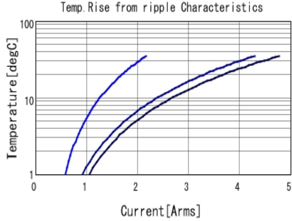
GRM31MR71E105KA01 Temp. rise ■ 100kHz ■ 500kHz ■ 1MHz
