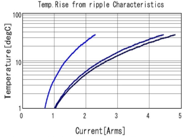
GRM31MR71C105KA01 Temp. rise ■ 100kHz ■ 500kHz ■ 1MHz
