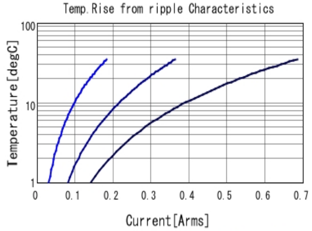
GRM31CR72E333KW03 Temp. rise ■ 30kHz ■ 100kHz ■ 300kHz
