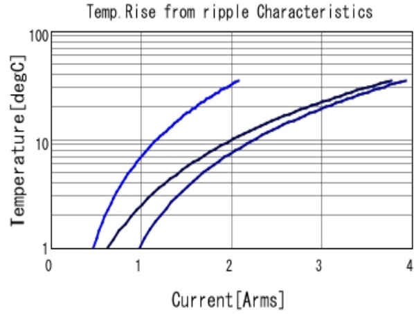
GRM31CR72A105KA01 Temp. rise ■ 100kHz ■ 500kHz ■ 1MHz
