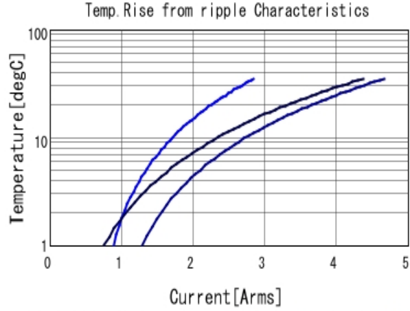
GRM31CR71H225KA88 Temp. rise ■ 100kHz ■ 500kHz ■ 1MHz
