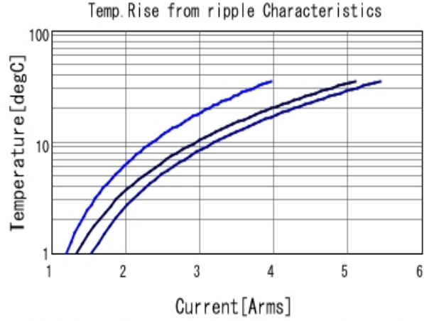
GRM31CR71E475KA88 Temp. rise ■ 100kHz ■ 500kHz ■ 1MHz
