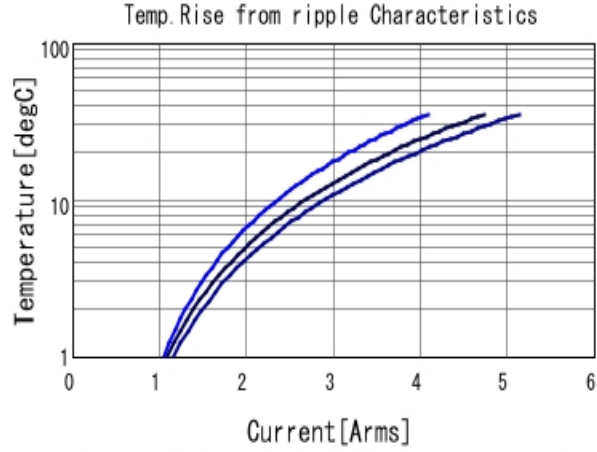
GRM31CR71C475KA01 Temp. rise ■ 100kHz ■ 500kHz ■ 1MHz
