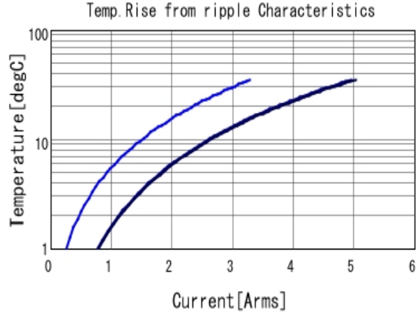
GRM31CR71C106KAC7 Temp. rise ■ 80kHz ■ 400kHz ■ 800kHz
