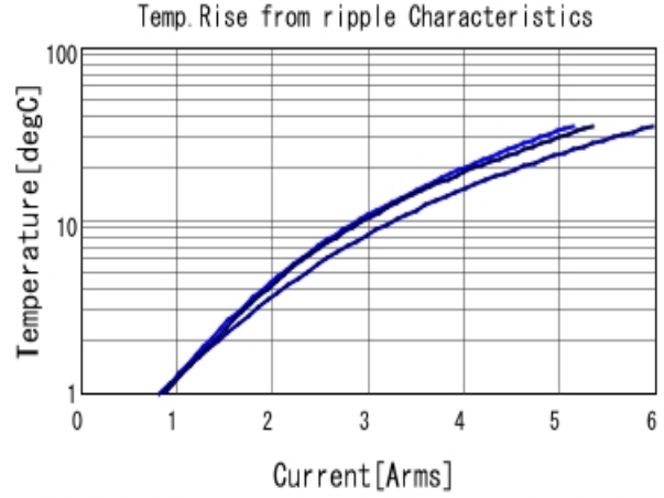
GRM31CR71C106KA12 Temp. rise ■ 100kHz ■ 500kHz ■ 1MHz
