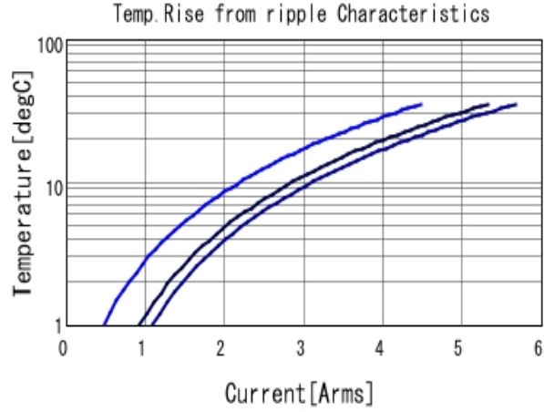
GRM31CR71A226KE15 Temp. rise ■ 80kHz ■ 400kHz ■ 800kHz
