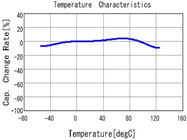
■ GRM31CR71A226KE15 C-Temp. capchange, DCO. 0V, ACO. 5V rm
