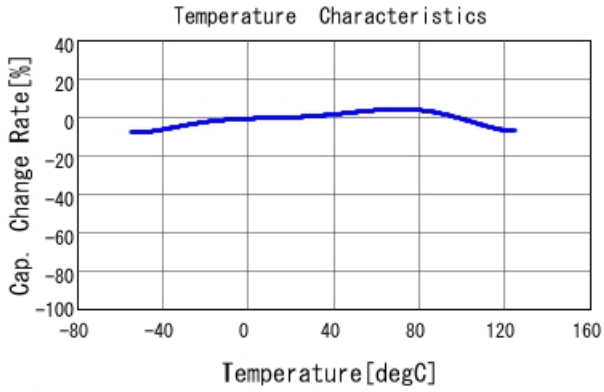
■ GRM31CR70J226ME19 C-Temp. capchange, DCO. 0V, ACO. 5Vrm
