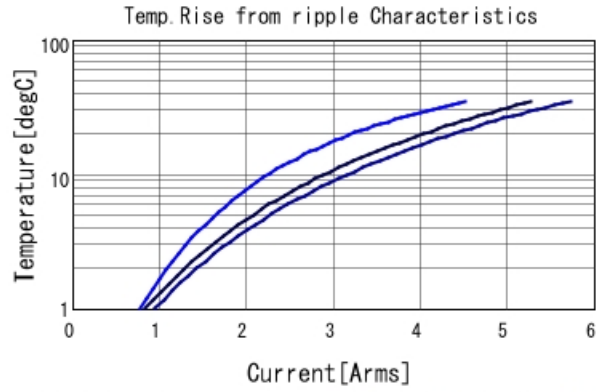
GRM31CR70J226ME19 Temp. rise ■ 100kHz ■ 500kHz ■ 1MHz
