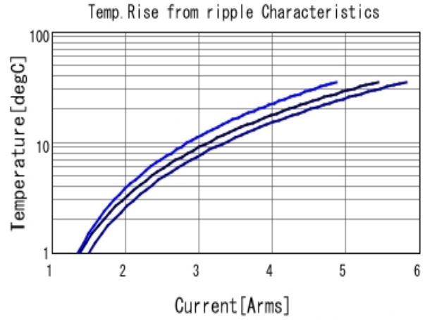
GRM31CR70J106KA01 Temp. rise ■ 80kHz ■ 400kHz ■ 800kHz
