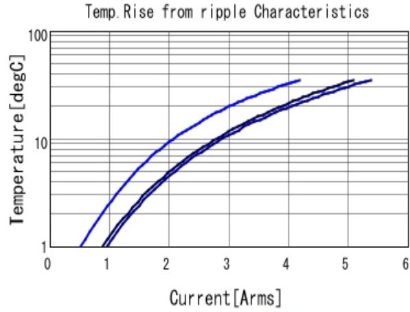
GRM31CR61H106KA12 Temp. rise ■ 100kHz ■ 500kHz ■ 1MHz
