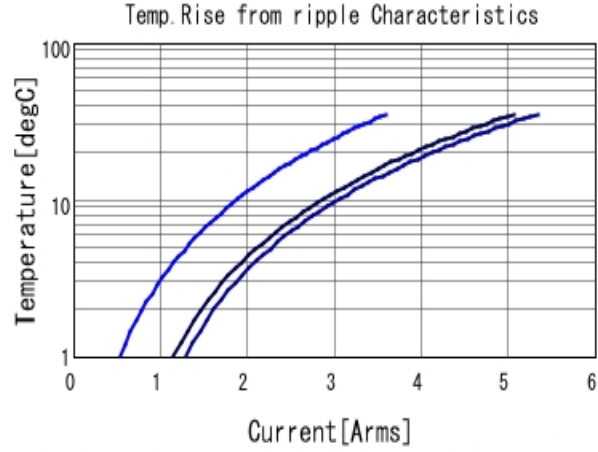
GRM31CR61E106KA12 Temp. rise ■ 80kHz ■ 400kHz ■ 800kHz
