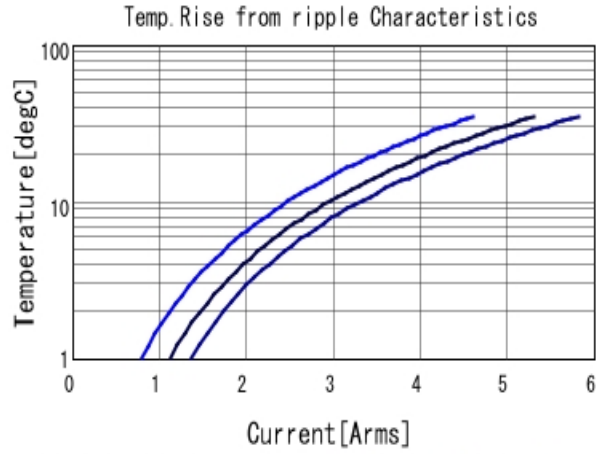
GRM31CR61C226KE15 Temp. rise ■ 80kHz ■ 400kHz ■ 800kHz
