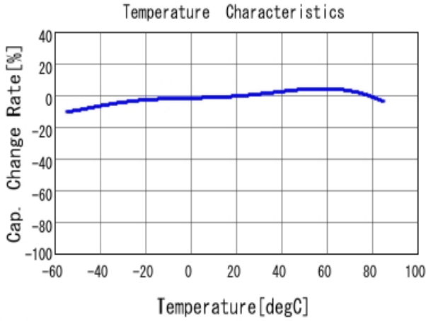
■ GRM31CR61C226KE15 C-Temp. capchange, DCO. 0V, ACO. 5V rm
