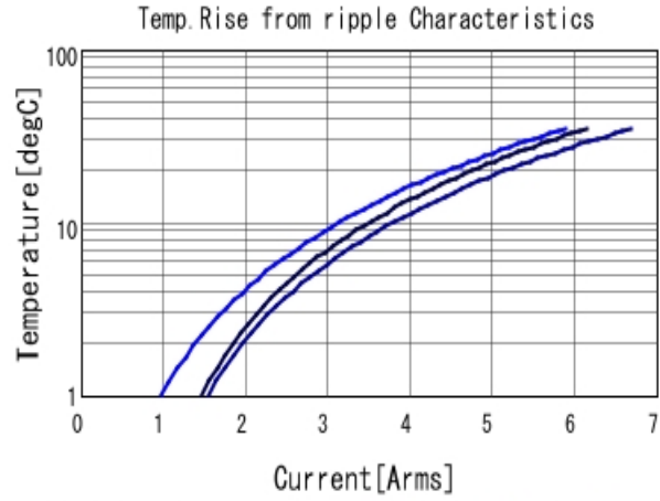
GRM31CR60J476ME19 Temp. rise ■ 60kHz ■ 300kHz ■ 600kHz
