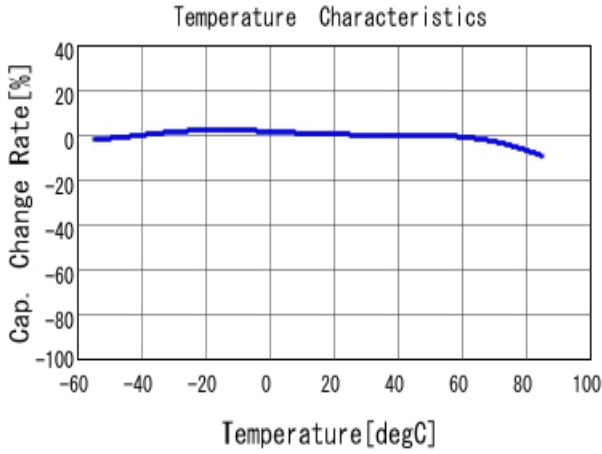
■ GRM31CR60J476ME19 C-Temp. capchange, DCO. 0V, ACO. 5V rm
