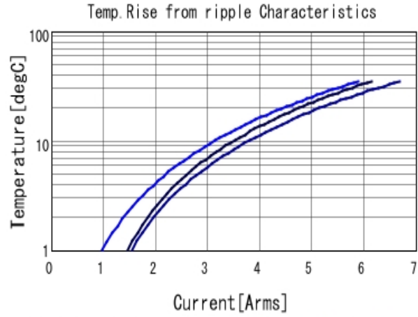
GRM31CR60J476KE19 Temp. rise ■ 60kHz ■ 300kHz ■ 600kHz
