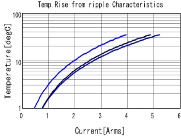
GRM31CC72A475KE11 Temp. rise ■ 100kHz ■ 500kHz ■ 1MHz
