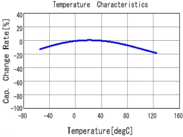
■ GRM31CC72A475KE11 C-Temp. capchange, DCO. 0V, ACO. 1Vrm
