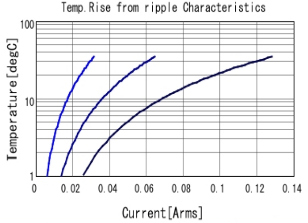
GRM31BR73A102KW01 Temp. rise ■ 30kHz ■ 100kHz ■ 300kHz
