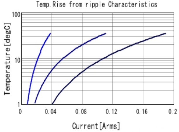
GRM31BR72J222KW01 Temp. rise ■ 30kHz ■ 100kHz ■ 300kHz
