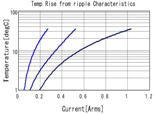
GRM31BR72E683KW01 Temp. rise ■ 30kHz ■ 100kHz ■ 300kHz
