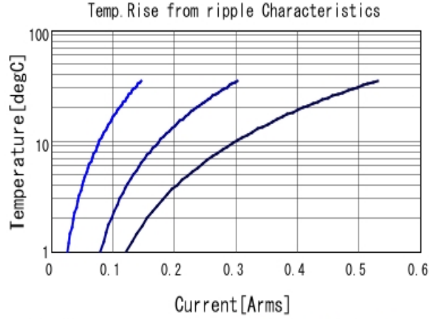
GRM31BR72E223KW01 Temp. rise ■ 30kHz ■ 100kHz ■ 300kHz
