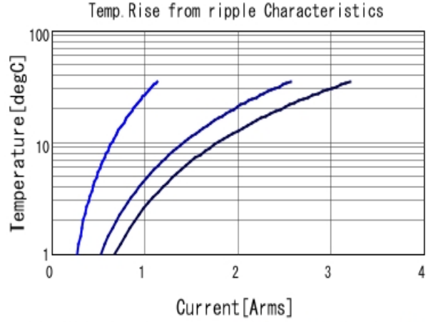
GRM319R71H334KA01 Temp. rise ■ 100kHz ■ 500kHz ■ 1MHz
