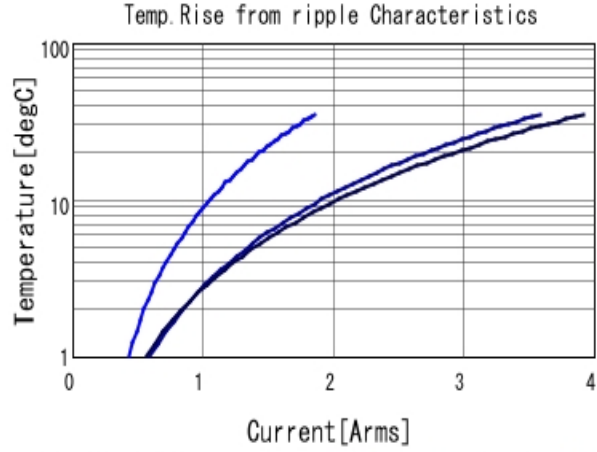
GRM319R71C105KAA3 Temp. rise ■ 100kHz ■ 500kHz ■ 1MHz
