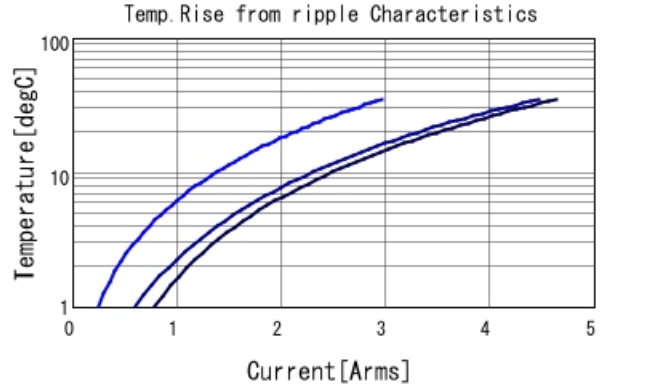
GRM319R61E475KA12 Temp. rise — 100kHz — 500
