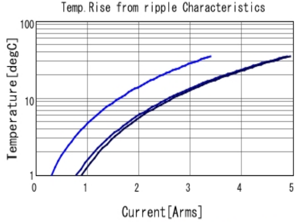
GRM319R61C106KE15 Temp. rise ■ 80kHz ■ 400kHz ■ 800kHz
