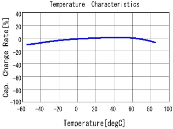
■ GRM319R61C106KE15 C-Temp. capchange, DCO. 0V, ACO. 5V rm
