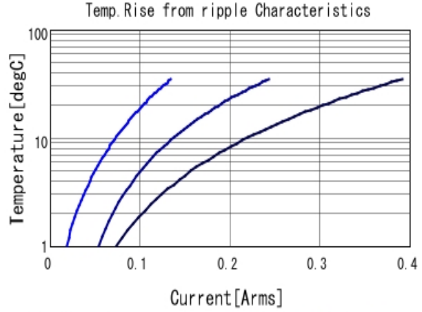
GRM21BR72E103KW03 Temp. rise ■ 30kHz ■ 100kHz ■ 300kHz
