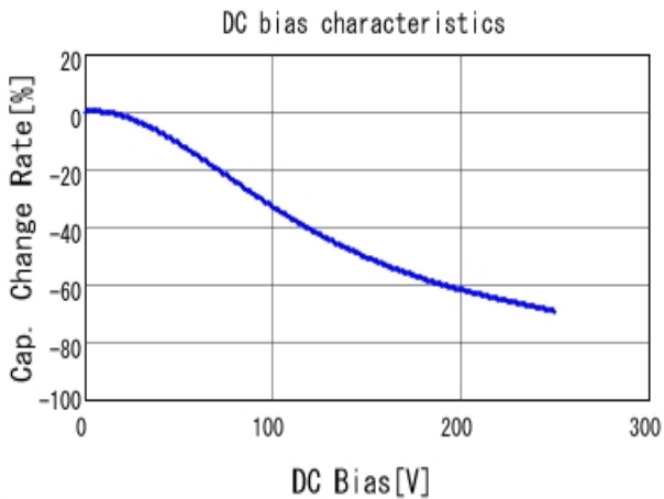
■ GRM21BR72E103KW03 C-DC bias capchange, 25.0degC, AC1V
