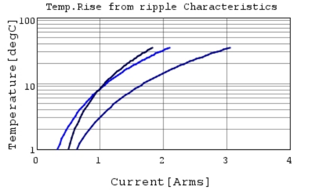
GRM21BR72A474KA73 Temp.rise — 200kHz —
