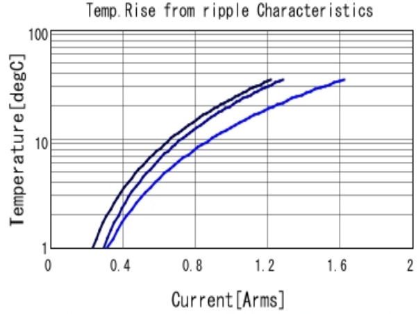
GRM21BR72A104KAC4 Temp. rise ■ 400kHz ■ 800kHz ■ 1MHz
