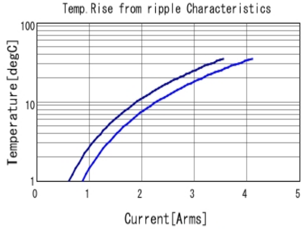
GRM21BR71H105KA12 Temp. rise ■ 500kHz ■ 1MHz
