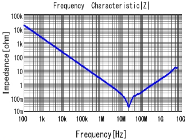
■ GRM21BR71H104KA01 |Z| DCOV, 25degC
