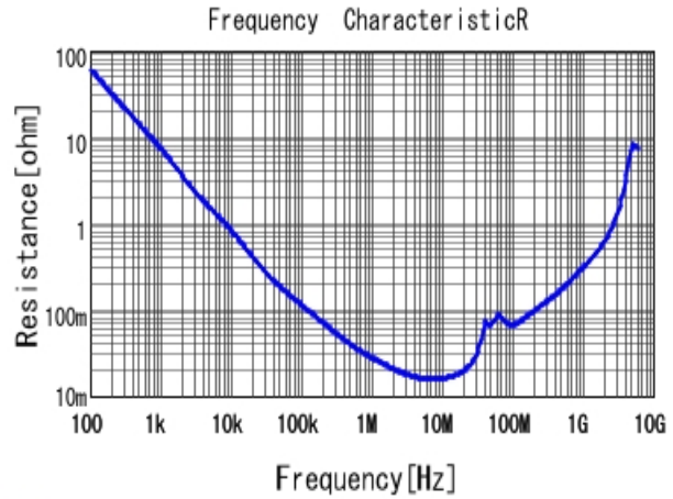
■ GRM21BR71H104KA01 R DCOV, 25degC
