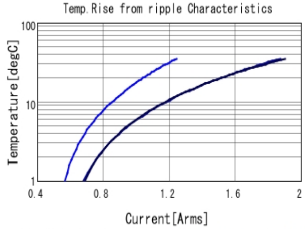
GRM21BR71H104KA01 Temp. rise ■ 400kHz ■ 800kHz ■ 1MHz
