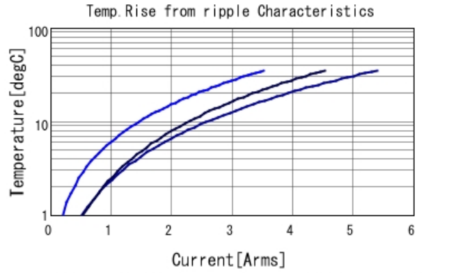
GRM21BR71E475KA73 Temp. rise — 100kHz — 500
